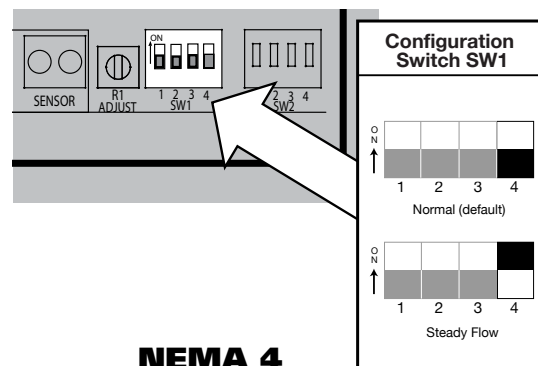
NEMA 4
